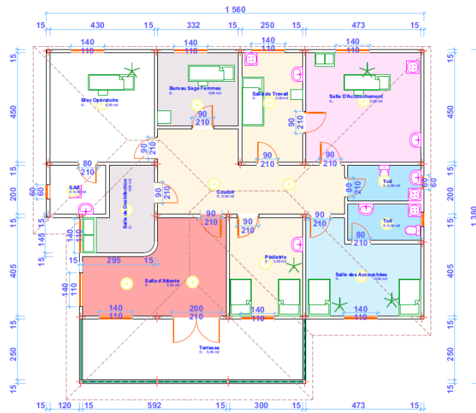
VUE EN PLAN ECH: 1/100
